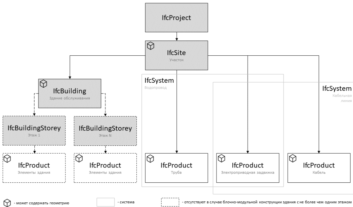
Рисунок 1.1 – Пространственная структура ЦИМ в формате IFC
